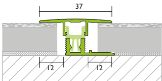
mit Erhöhungsteil
