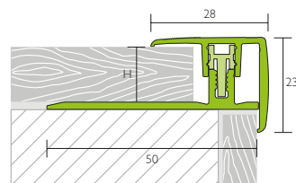
mit Erhöhungsteil
