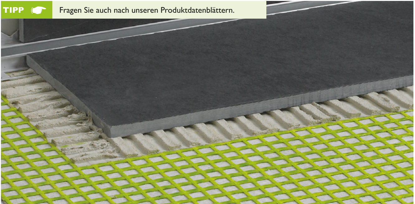
PROSECUREfibretec 2.0 Armierungs- und Entkopplungsmatte
