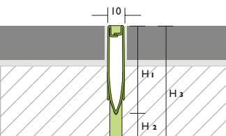
Oberflächenbündige Ausbildung: Optisch verstärkt dargestellt.
