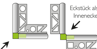
Eckstück als Außenecke
