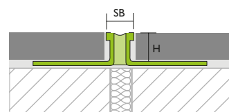
Oberflächennahe Ausbildung: Optisch verstärkt dargestellt.
