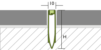
Oberflächenbündige Ausbildung: Optisch verstärkt dargestellt.
