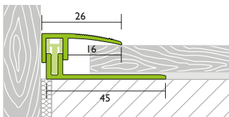
mit Erhöhungsteil
