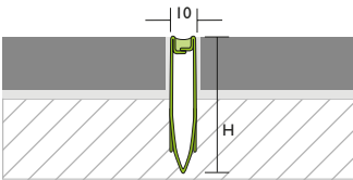
Oberflächennahe Ausbildung: Optisch verstärkt dargestellt.
