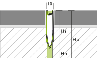
Oberflächennahe Ausbildung: Optisch verstärkt dargestellt.
