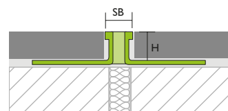
Oberflächenbündige Ausbildung: Optisch verstärkt dargestellt.
